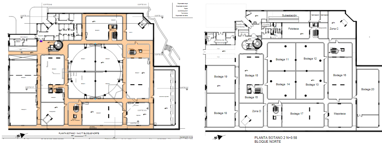
A la izquierda: planta bloque norte nivel -1. A la derecha: planta bloque norte nivel-2. Áreas de custodia documental
