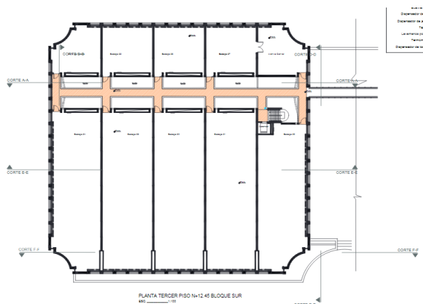
Planta bloque sur. Nivel 3. Áreas de custodia documental
