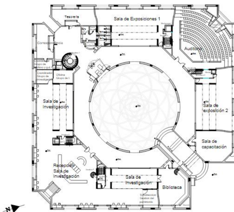
PLANTA PRIMER PISO N+7.67 BLOQUE NORTE
